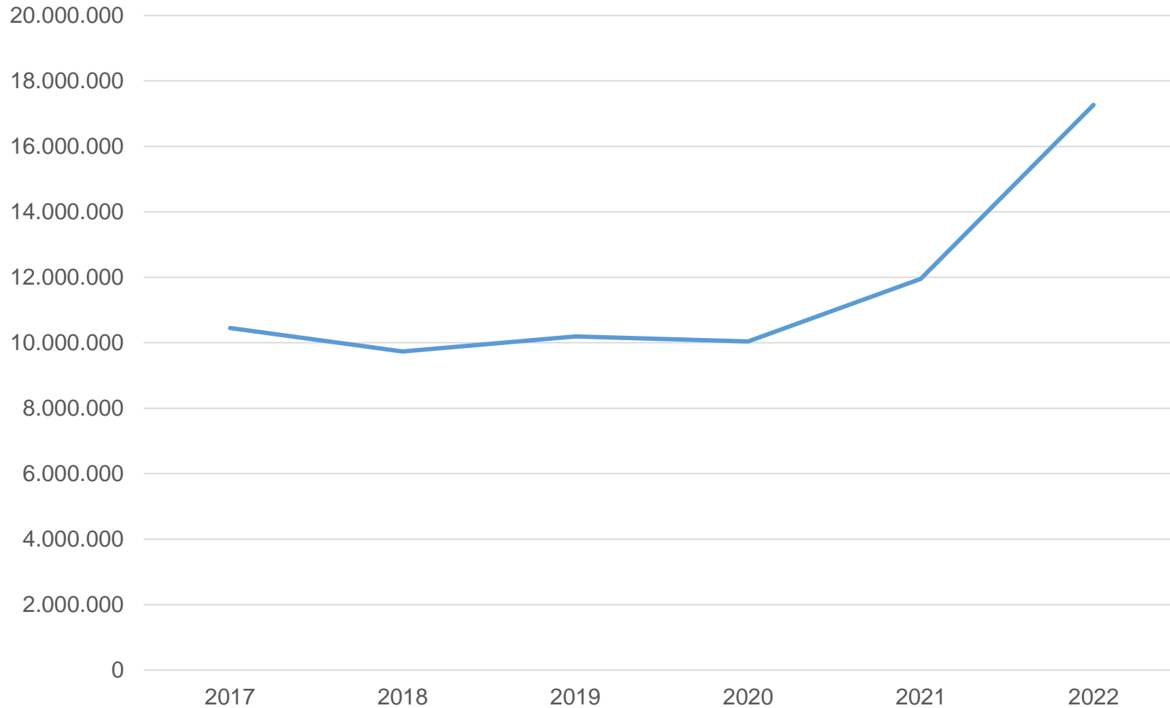
Gewerbesteuereinnahmen Renningen
